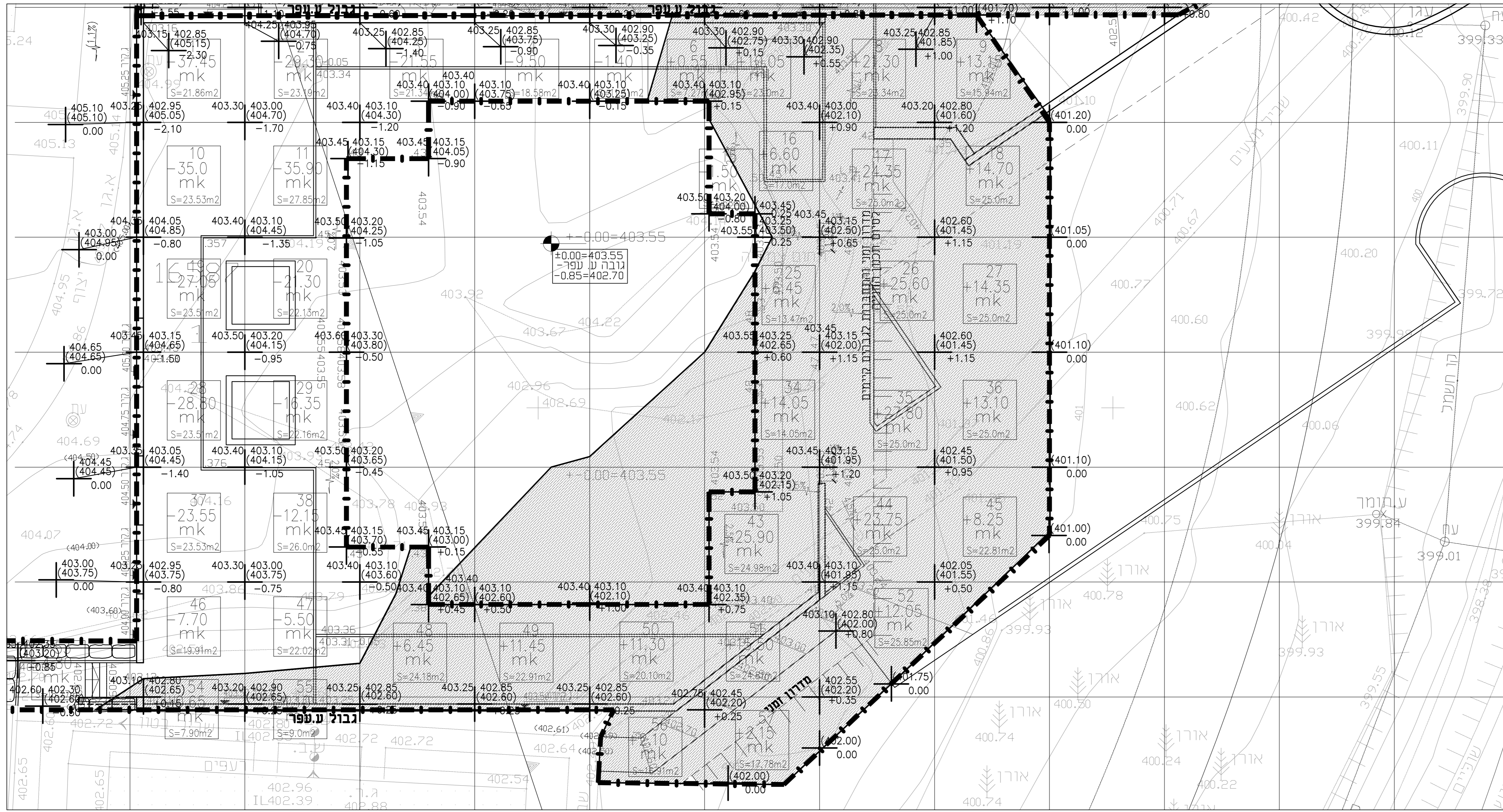
תכנית עבודות עפר-פיתוח קנ"מ: 1:100
