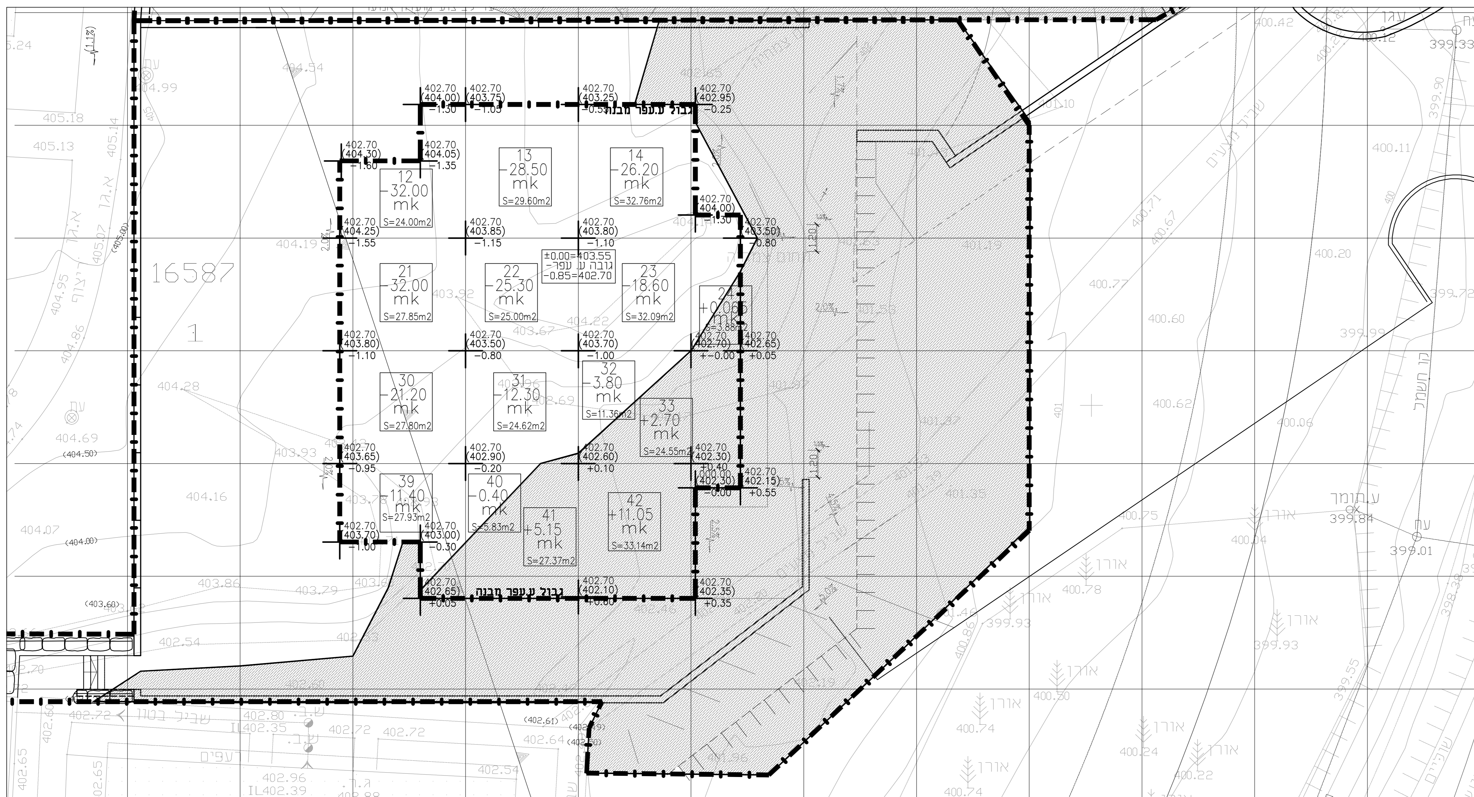
תכנית עבודות עפר-מבנה קנ"מ: 1:100
